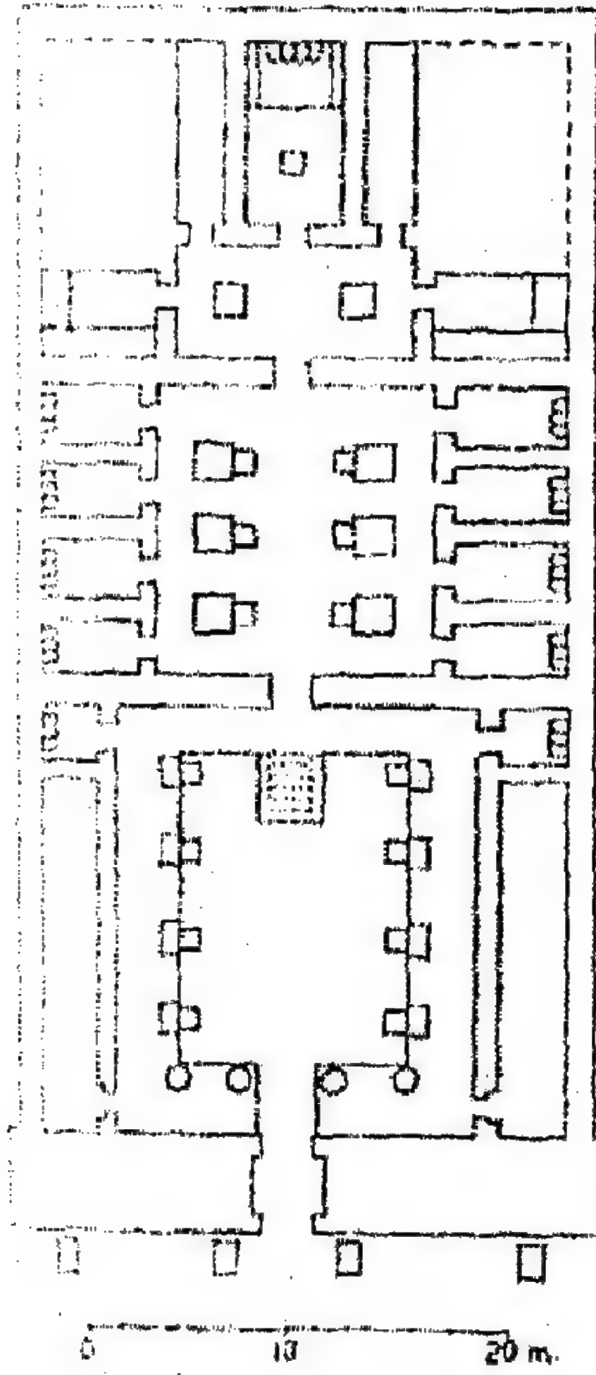
خريطة معبد " جرف حسين " .
